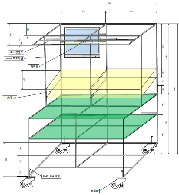
조립 작업대
